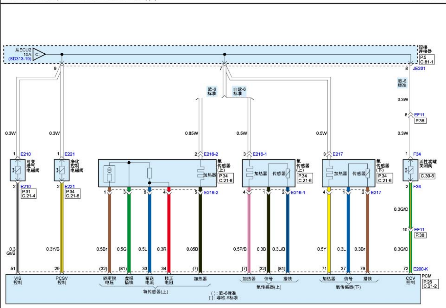
发动机控制系统(G4FG : GAMMA 1.6L MPI)(4)
